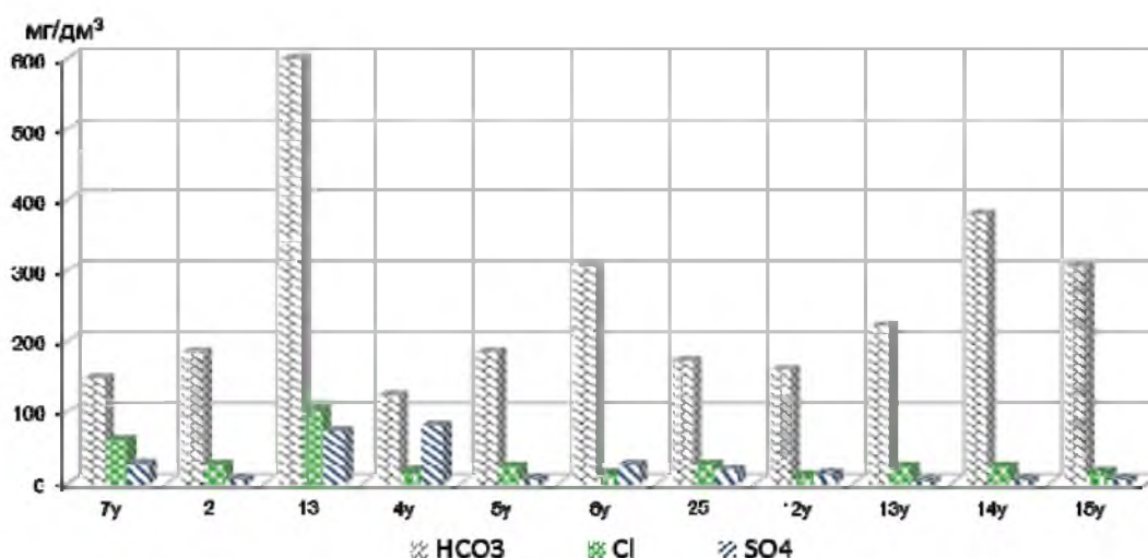
Рис. 7. Аніонний склад ґрунтових вод за свердловинами (межиріччя Західного Бугу і Прип'яті, 2015 р.)
