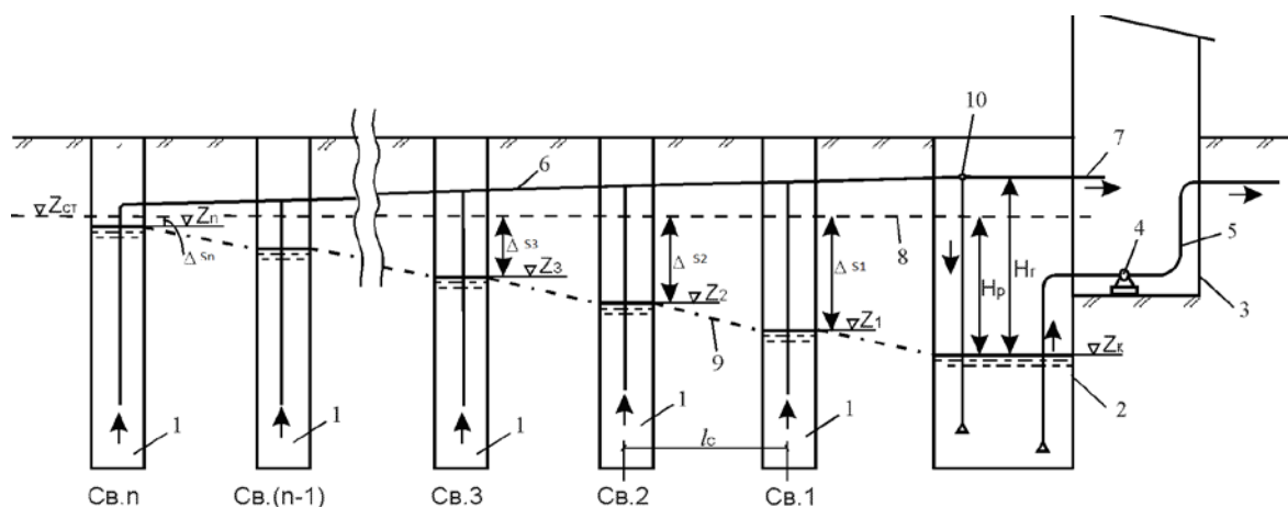
Рис. 1. Схема відведення води від групи з n свердловин сифонним збірним водоводом: 1 – водозабірні свердловини; 2 – водоприймальний збірний колодезь; 3 – насосна станція; 4 – горизонтальний відцентровий насос; 5 – напірний трубопровід; 6 – сифонний збірний водовід; 7 – труба до вакуум-насоса; 8 – лінія статичного рівня води у водоносному пласті; 9 – н'єзометрична лінія в сифонному збірному водоводі; 10 – найвища точка сифонного водоводу
